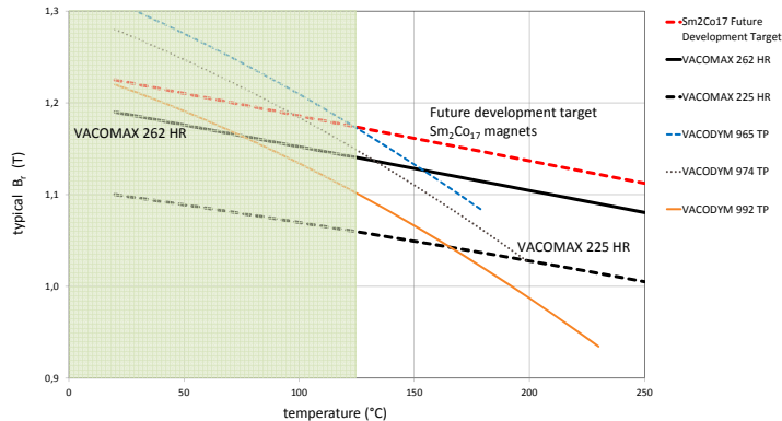
Temperaturabhängigkeit der Remanenz verschiedener VACOMAX und VACODYM Legierungen
